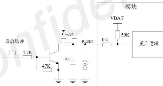
图 12: 复位推荐电路
