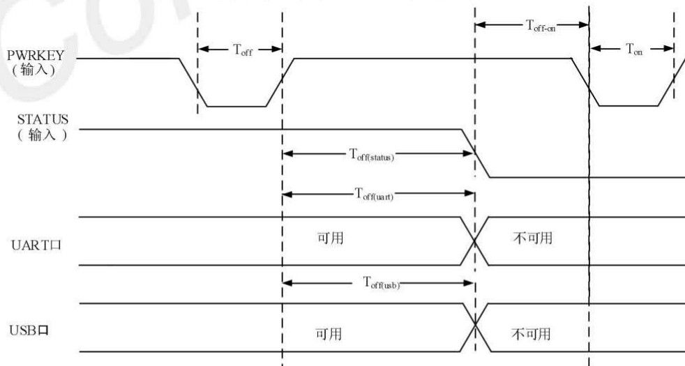
图 11: PWRKEY 关机时序
