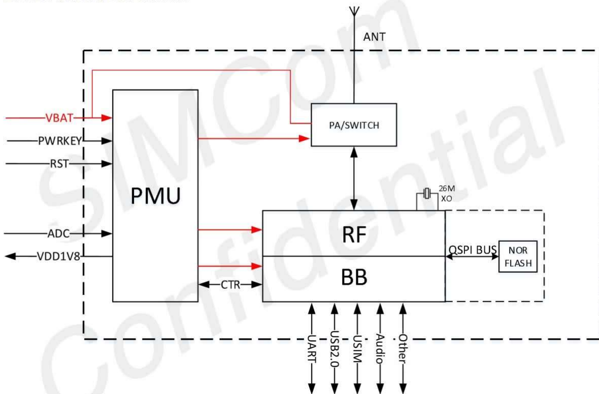
图 1：模块框图
