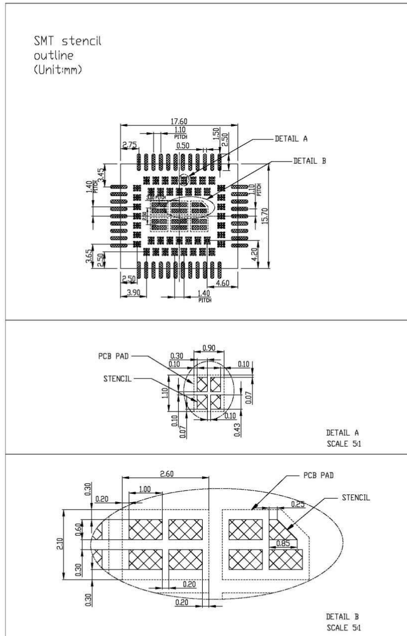
图 5: 推荐钢网尺寸 (单位: 毫米)
