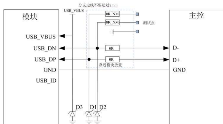
图 17: USB 连接图
