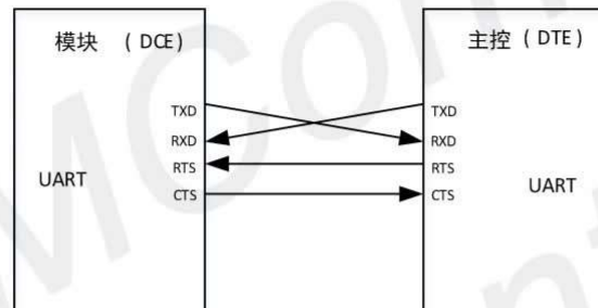
图 13: 串口连接图（全功能模式）
