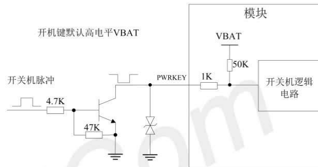
图 9：开机参考电路
