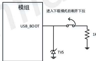
图 18: USB_BOOT 连接图
