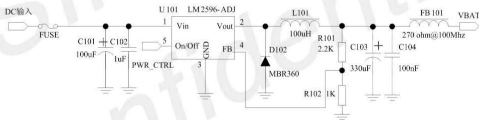
图 8：开关电源推荐电路
