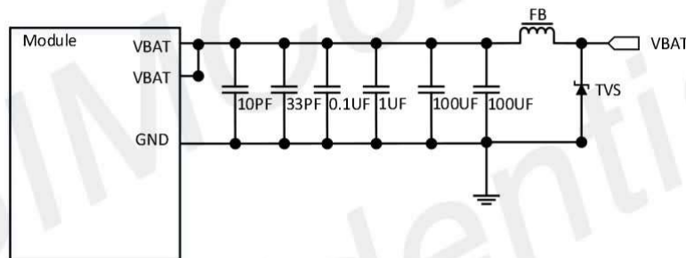
图 6: VBAT 输入参考电路
