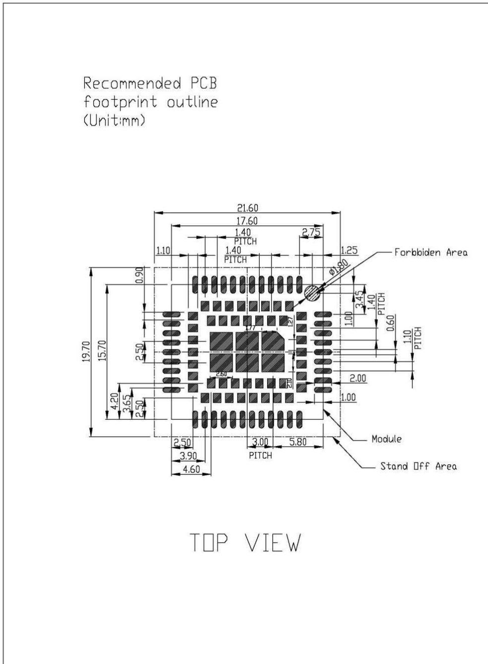
图 4: 推荐 PCB 封装尺寸 (单位: 毫米)
