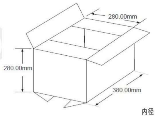
图 32: 托盘大卡通箱尺寸图
