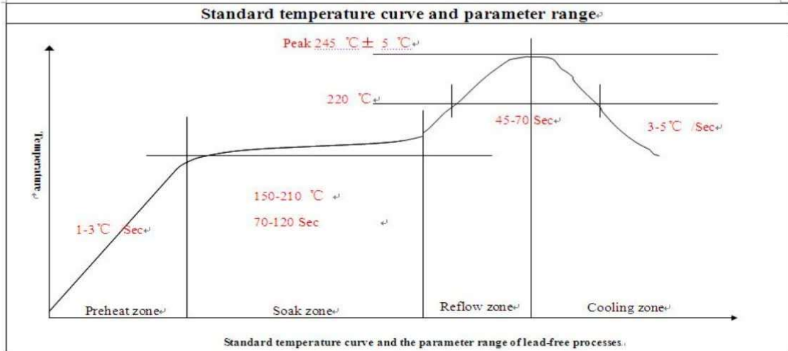
图 28: 推荐焊接炉温曲线图 (无铅工艺)
