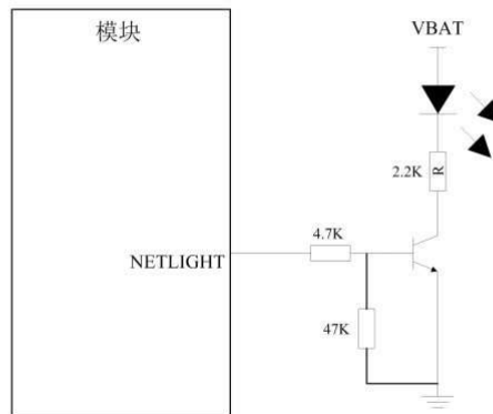
图 23: NETLIGHT 参考电路
