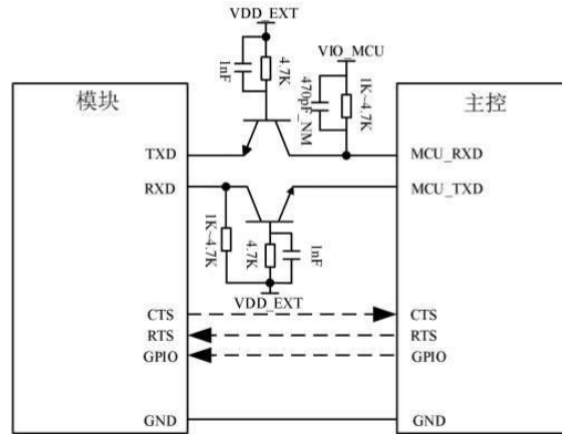
图 15: 三极管电平转换电路
