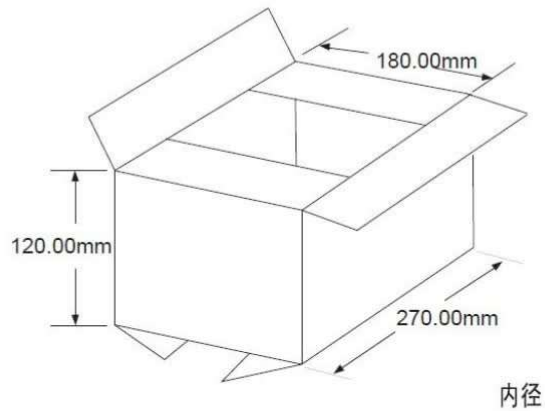
图 31: 托盘小卡通箱尺寸图
