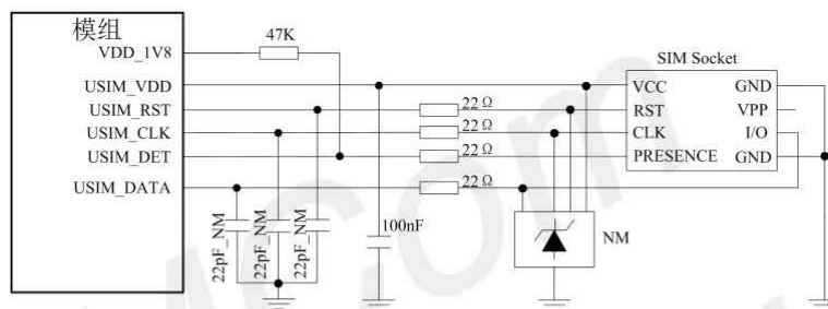
图 21: USIM 接口推荐电路(8PIN)
