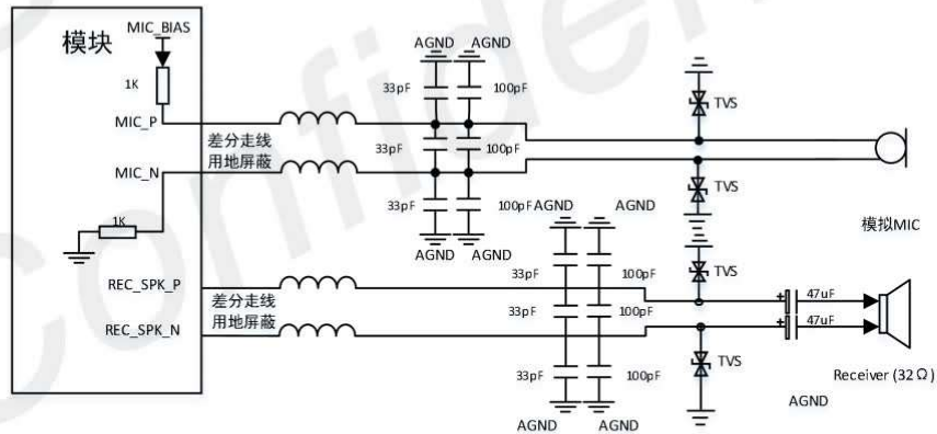
图 22: 模拟音频接口推荐电路
