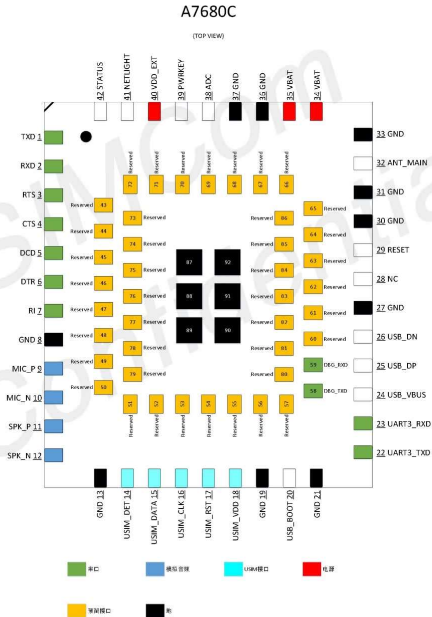
图 2: 模块引脚图(正面视图)
