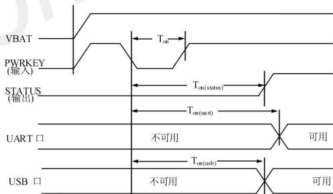
图 10：PWRKEY 开机时序
