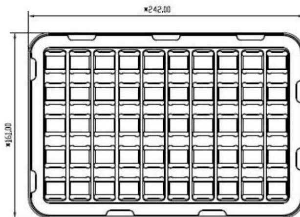
图 30: 托盘尺寸图
