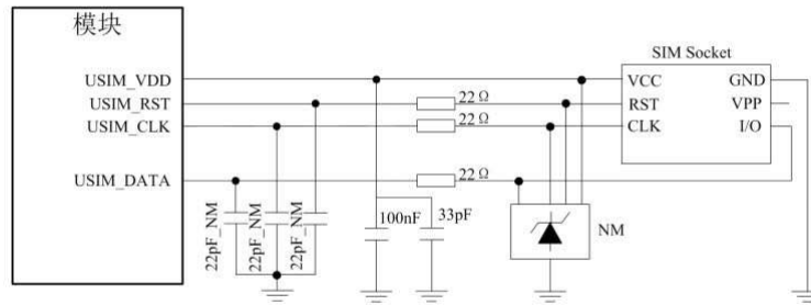
图 20: USIM 接口推荐电路
